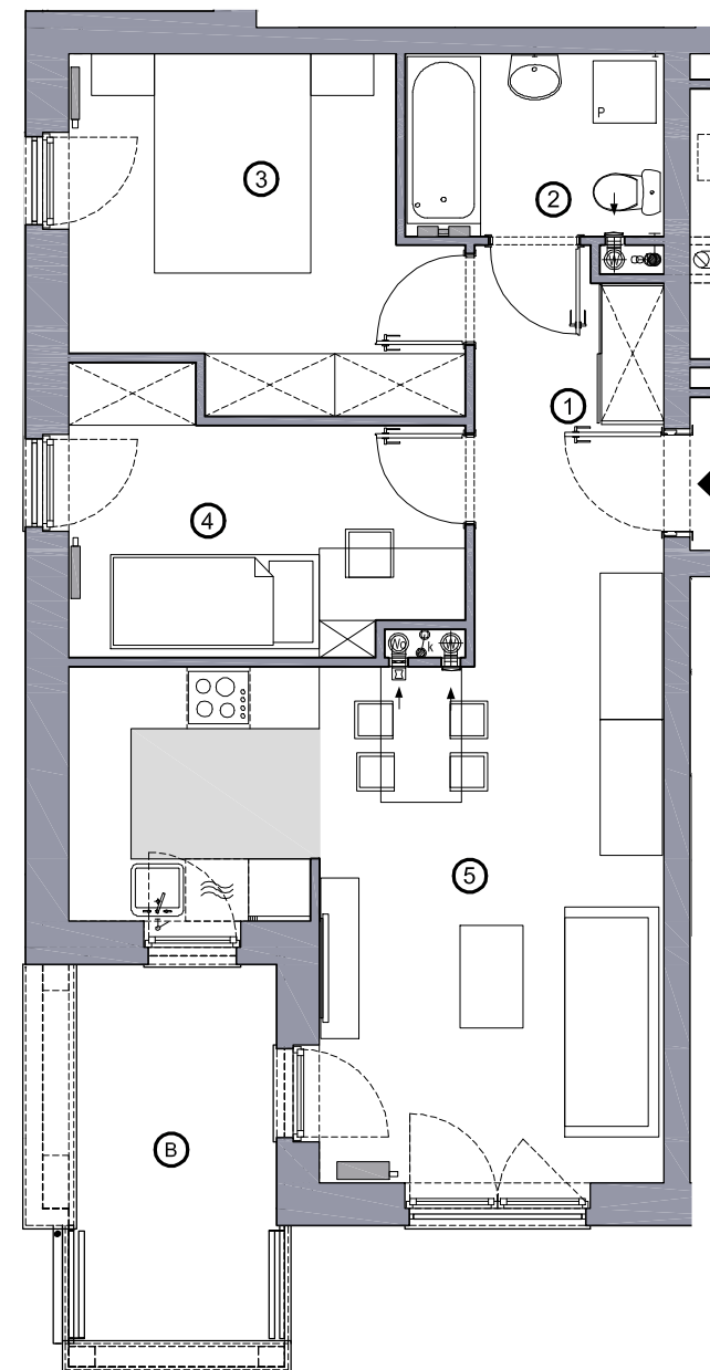
RZUT MIESZKANIA
