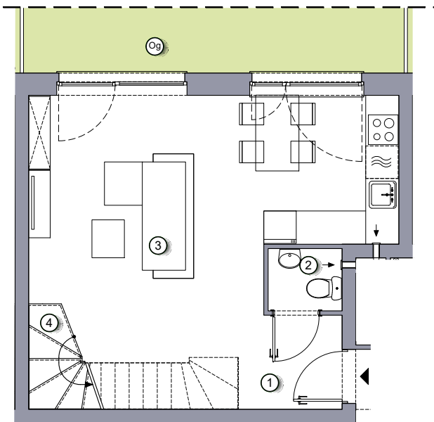
Rzut parteru
