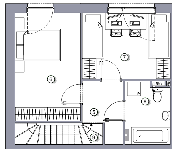
Rzut 1 piętra
