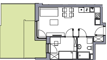
Rzut ogrodu
