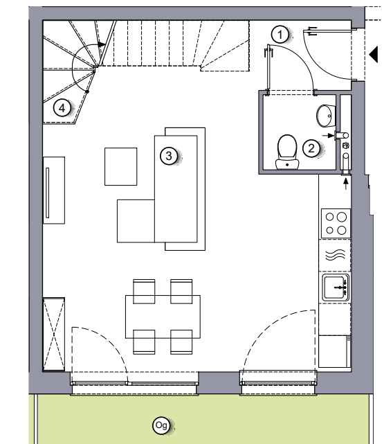
Rzut parteru
