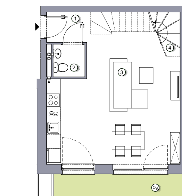
Rzut parteru
