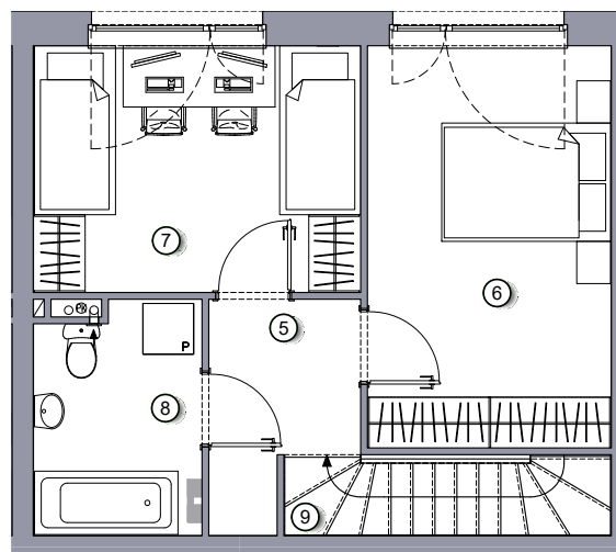
Rzut 1 piętra
