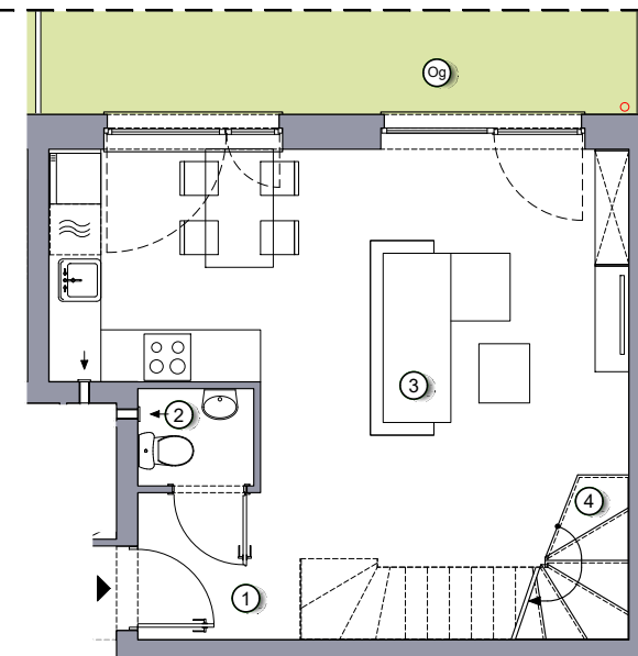
Rzut parteru
