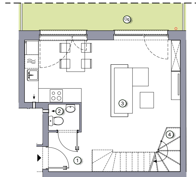
Rzut parteru
