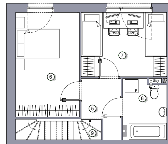
Rzut 1 piętra
